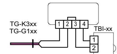
Abb. 6: Anschluss eines externen, separaten Fühlers und TBI-xx Potentiometer als Sollwertversteller
