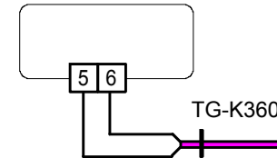
Abb. 7: Anschluss des Begrenzungsfühlers
