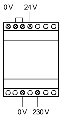
Fig. 1 Inkoppling för 24 V
