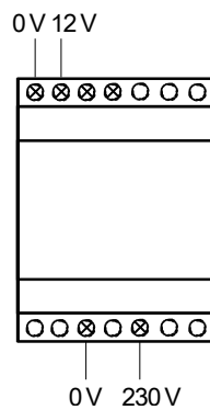
Fig. 2 Inkoppling för 12 V
