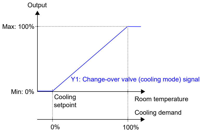
Fig. 2-7 Fonctionnement pour le mode Chauffage/Refroidissement (change-over) lorsque le régulateur est en mode refroidissement.
