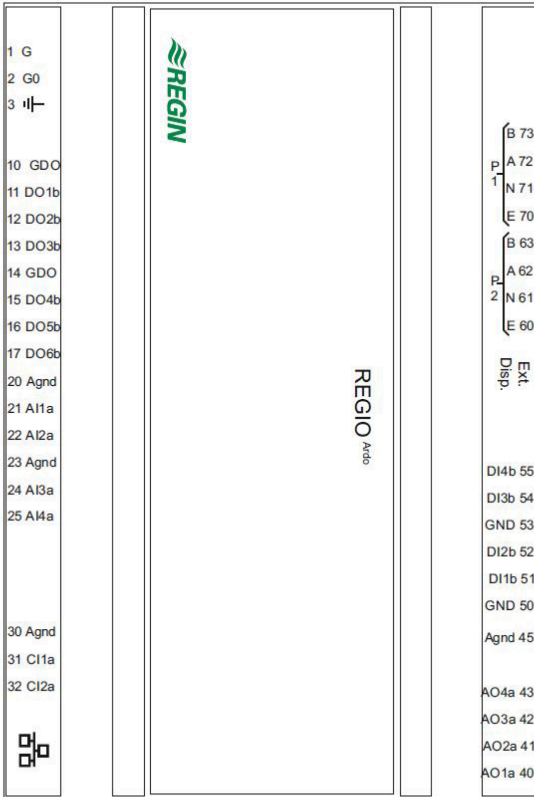
Fig. 7-1 Visual des raccordements du régulateur.
