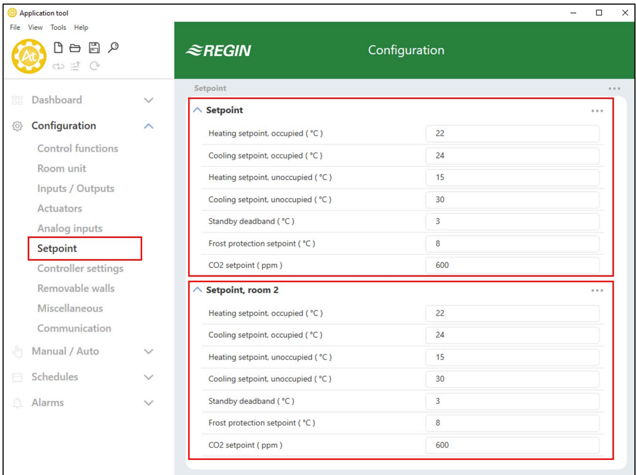
Fig. 2-42 Exemple du paramétrage de la zone 2 dans Application tool.
