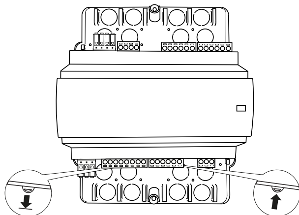
Fig. 9-3 Clipser l'automate sur le socle.
