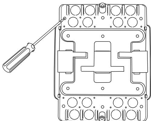
Fig. 9-2 Fixer le socle sur le mur.
