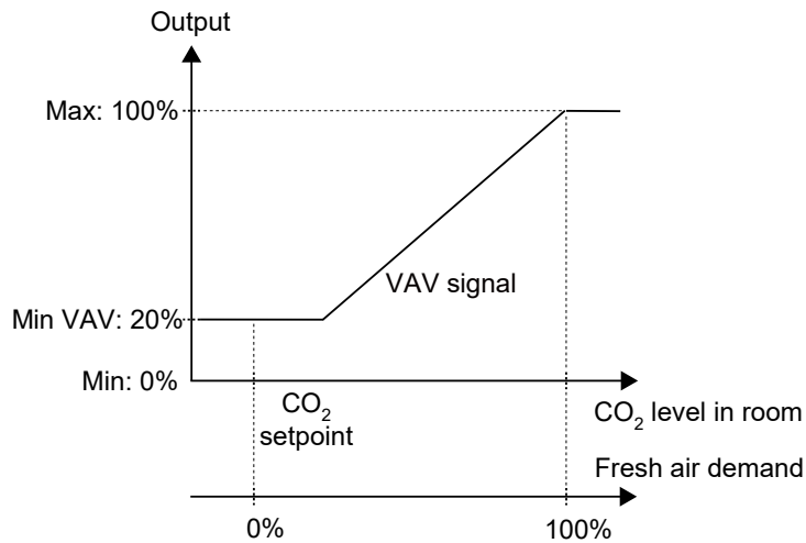
Fig. 2-43 Fonctionnement de régulation CO 2 .
