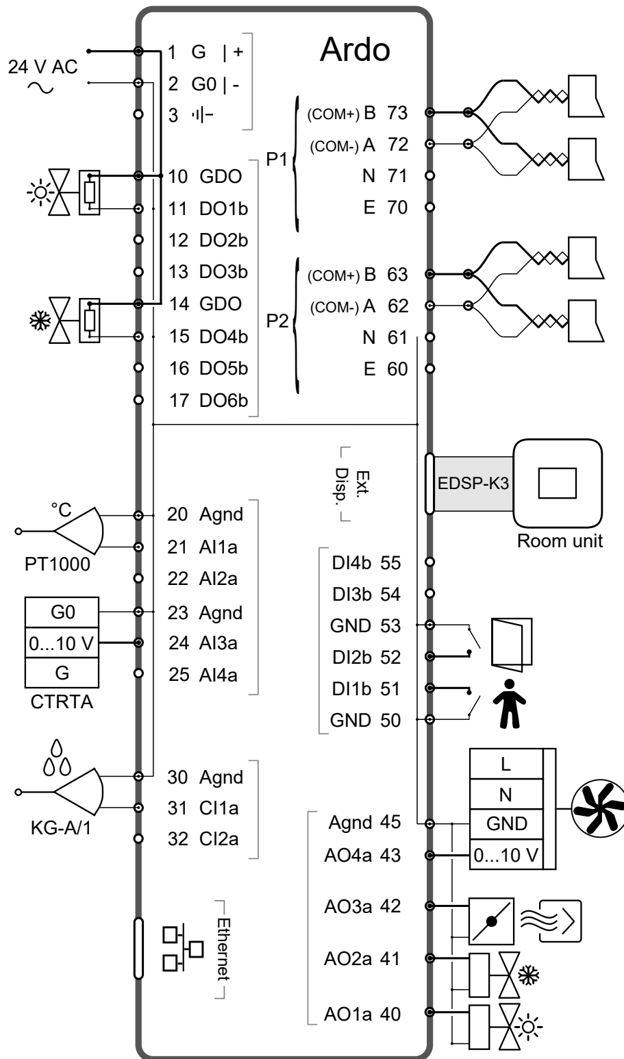
Fig. 7-2 Schéma de raccordement montrant un exemple d'utilisation des borniers de l'automate.
