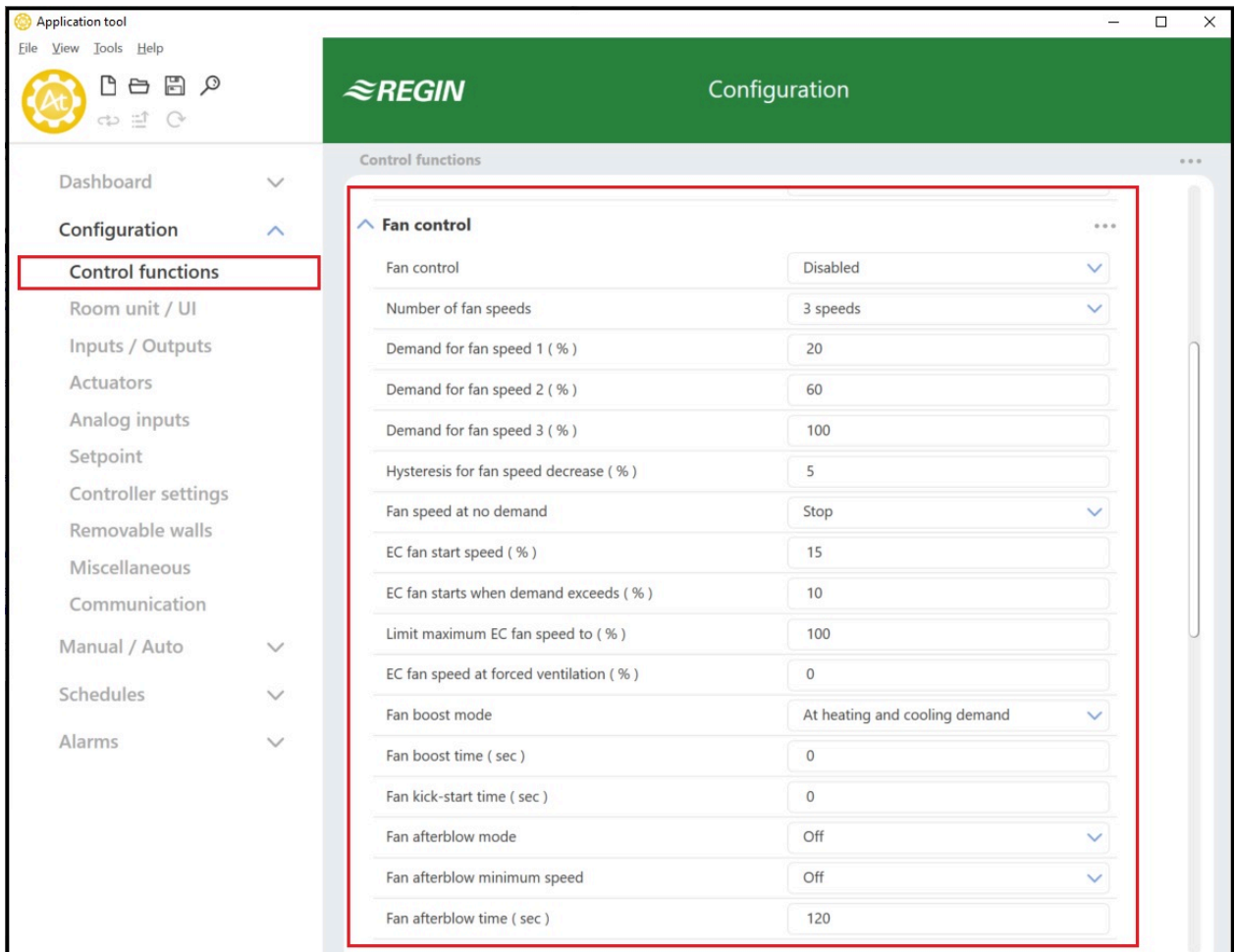
Fig. 2-29 Paramètres de la commande ventilateur 3 vitesses dans Application tool.
