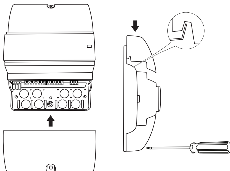
Fig. 9-4 Fixer et sécuriser les protège-borniers.
