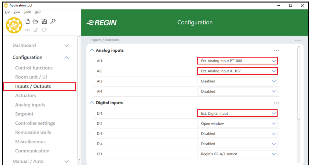
Fig. 4-2 Configuration des entrées du régulateur dans Application Tool.
