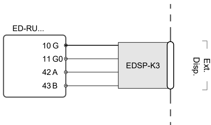
Fig. 7-3 Schéma de raccordement pour l'unité d'ambiance ED-RU-...
