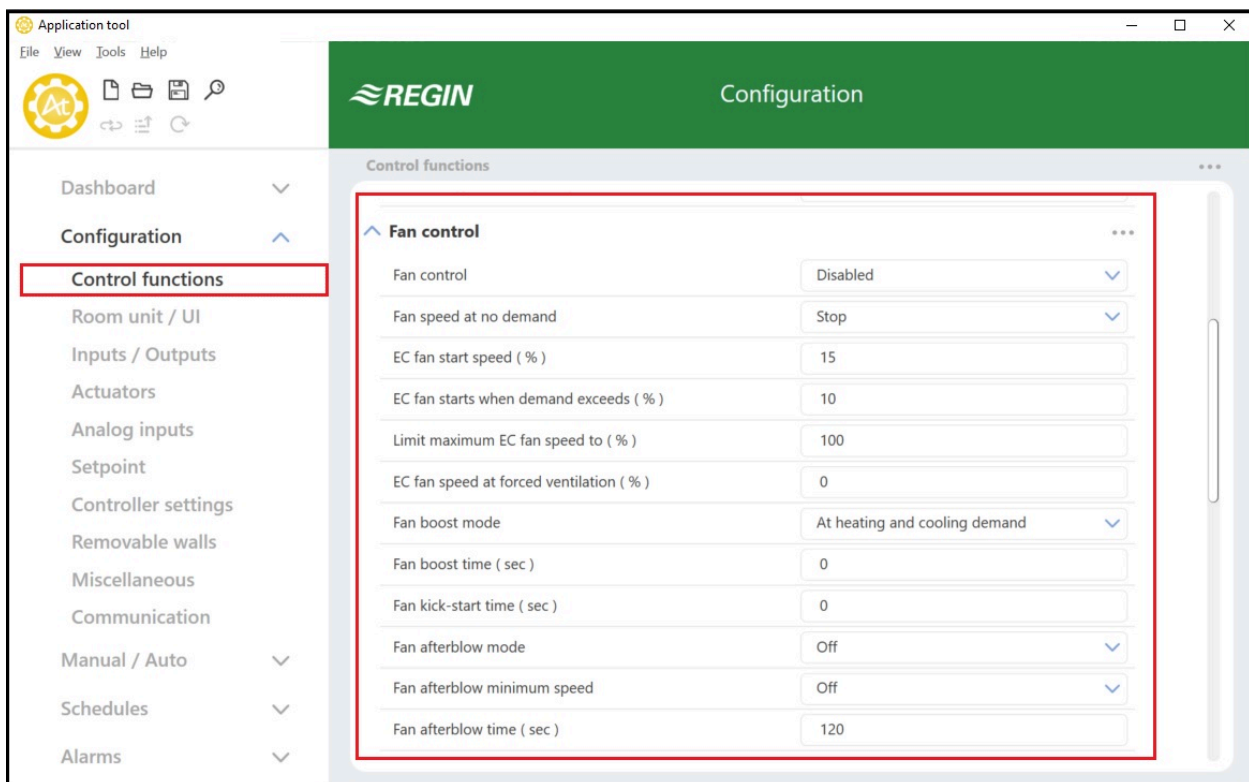
Fig. 2-26 Paramètres de configuration du contrôle de ventilateur EC dans Application tool.
