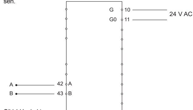
Bild 1 Verdrahtung
