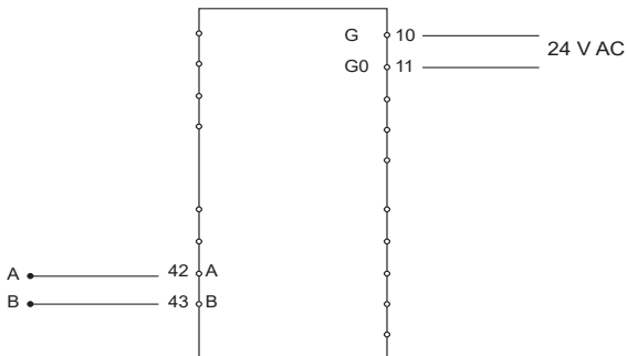
Figura 1 Cablaggio
