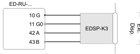
Figura 2 Cablaggio con un cavo EDSP-K3
