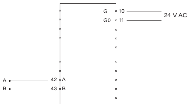
Bild 1 Verdrahtung
