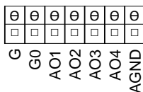
Figur 2 Inkopplingsschema
