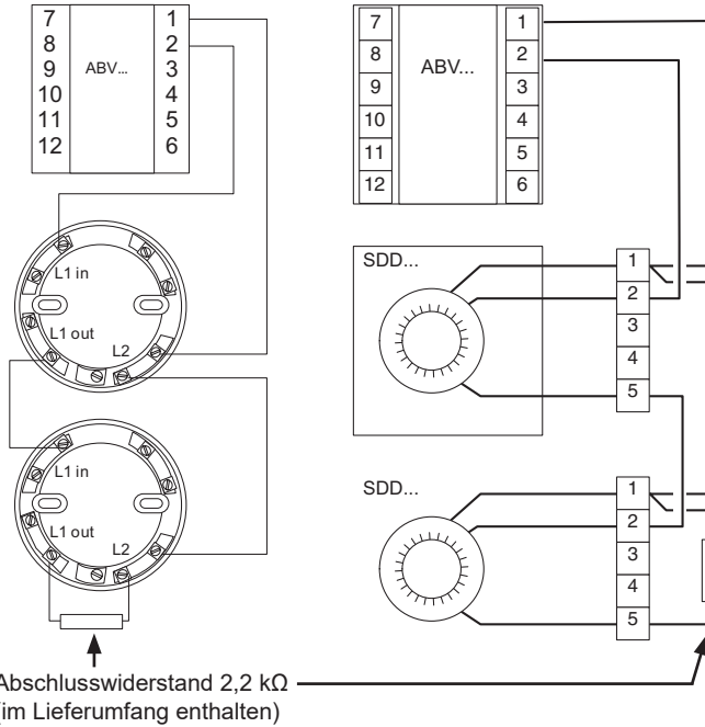
Abb. 2: Verdrahtung ABV(24)-S-300/D Verdrahtung ABV(24)-S-300/D und SDD... und S65...
