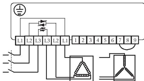
Schéma 1 : Raccordement de la tension d'alimentation et de la charge
