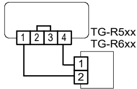
Abb. 2: Anschluss des Raumtemperaturfühlers TG-R5xx oder TG-R6xx bei Verwendung des internen Sollwertes
