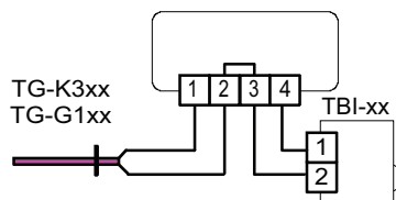
Abb. 6: Anschluss eines externen, separaten Fühlers und TBI-xx Potentiometer als Sollwertversteller
