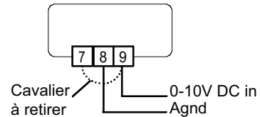
Schéma 8 : Raccordement pour un signal de commande externe
