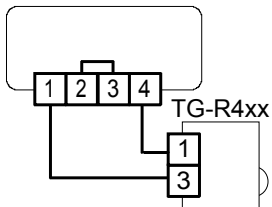
Abb. 3: Anschluss des TG-R430 als externer Fühler und Sollwertversteller bei Raumregelung.
