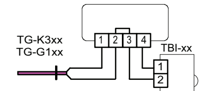
Schéma 6 : Raccordement en cas de sonde séparée externe et d'un potentiomètre TBI-xx comme réglage de consigne
