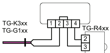
Abb. 5: Anschluss eines externen, separaten Fühlers und TG-R4XX lediglich als Sollwertversteller
