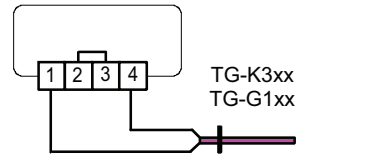
Bild 4 Anschluss eines Fußboden oder Kanalfühlers bei Verwendung des internen Sollwertes.
