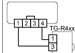
Fig. 3 Raccordement de la sonde d'ambiance externe TG-R430 et réglage de consigne en ambiance
