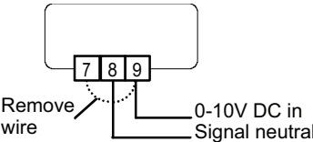
Bild 8 Anschluss bei externem Stellsignal
