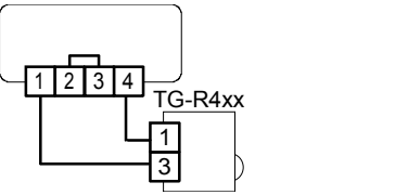
Bild 3 Anschluss des TG-R430 als externer Fühler und Sollwertversteller bei Raumregelung.
