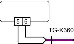
Bild 7 Verdrahtung des Begrenzungsfühlers
