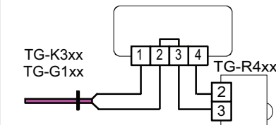
Fig. 5 Raccordement en cas de sonde séparée externe et d'une TG-R4xx comme réglage de consigne seulement
