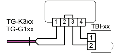
Bild 6 Anschluss eines externen, separaten Fühlers und TBIxx Potentiometer als Sollwertversteller
