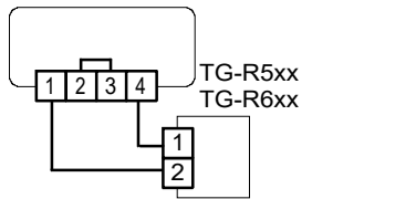
Bild 2 Anschluss des Raumtemperaturfühlers TG-R5xx oder TG-6Rxx bei Verwendung des internen Sollwertes
