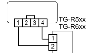
Fig. 2 Raccordement de la sonde d'ambiance TG-R5xx ou TG-R6xx en cas de fonctionnement avec une consigne interne
