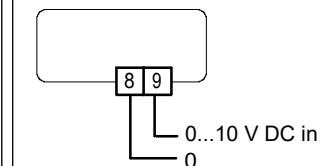
Abb. 2: Anschluss bei externem Stellsignal
