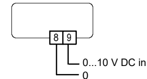
Figur 2: Inkoppling av styrsignal
