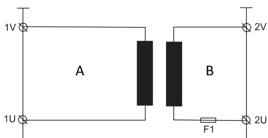
Fig. 1 A = Primaire (entrée), B = Secondaire (sortie)
