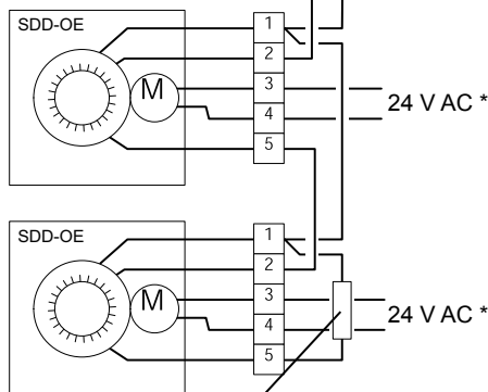
Inkoppling av reläfunktion
