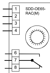
Figur 2. Inkoppling. Reläet visat i larmläge.
