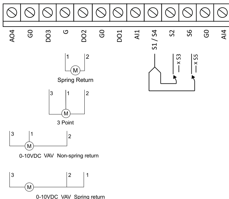
Figur 4-6 Ställdon och ändlägesbrytare
