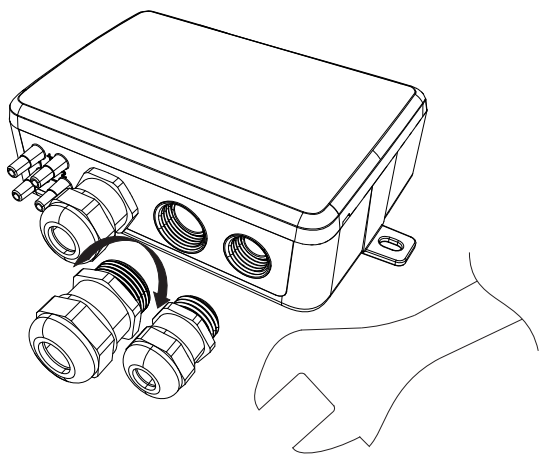
Figur 4-13 Installera kabelgenomföringar
