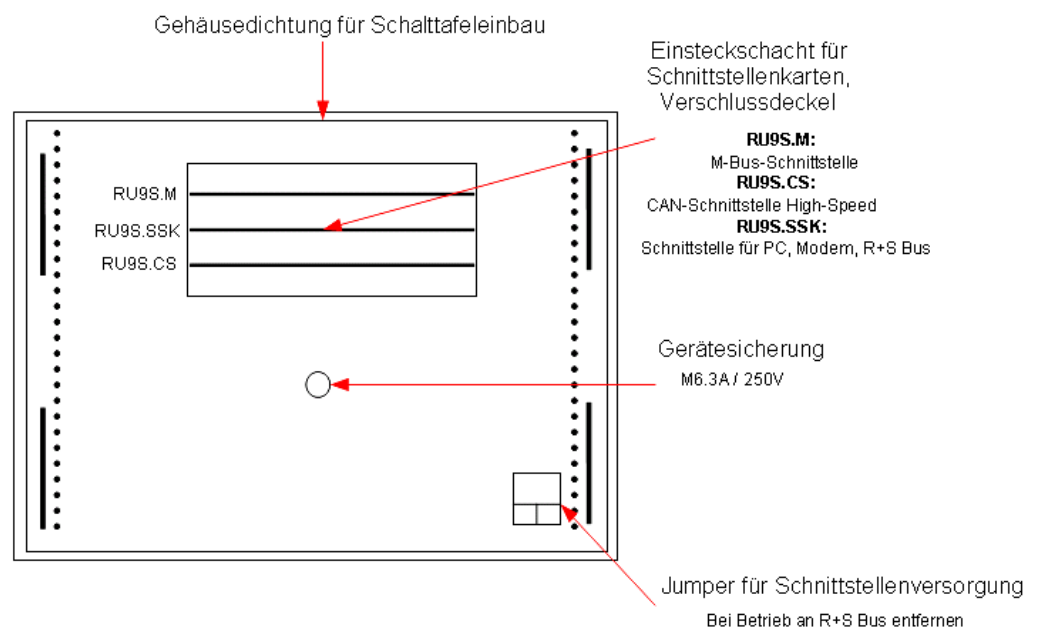
Abb. 3: Rückansicht
