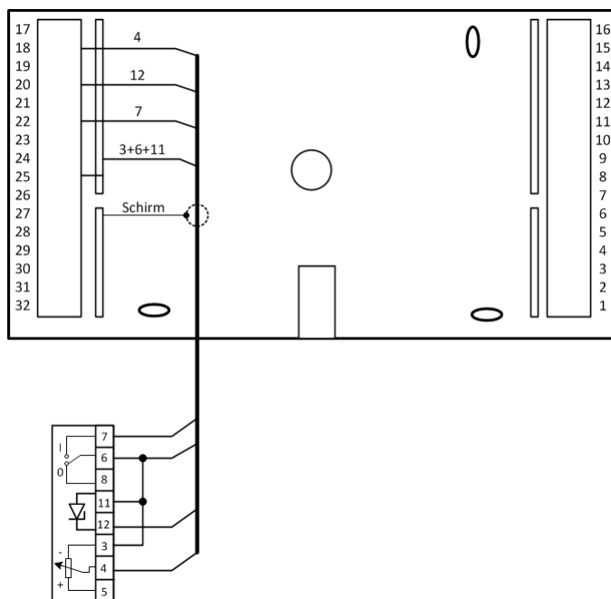
Abb. 13: Anschluss analoger Fernbedienungen
