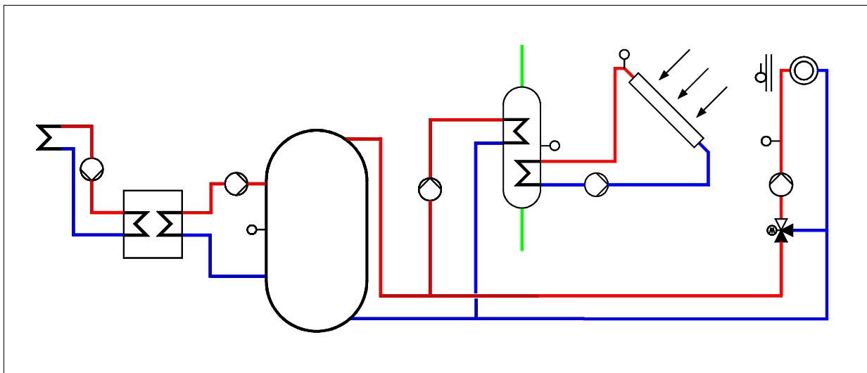
Schema 12: 1 Wärmepumpe (mit stetiger Ansteuerung) und Pufferspeicher, 1 Brauchwasser-kreis mit Ladepumpe zur Heizwasserladung und Solarladekreis, 1 gemischter Heizkreis
