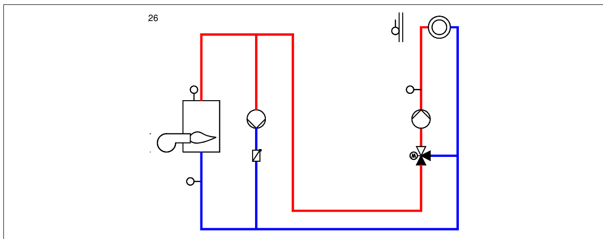
Schema 26: 1 Kessel (1- oder 2-stufig) mit Rücklauftemperaturbegrenzung, 1 gemischter Heizkreis
