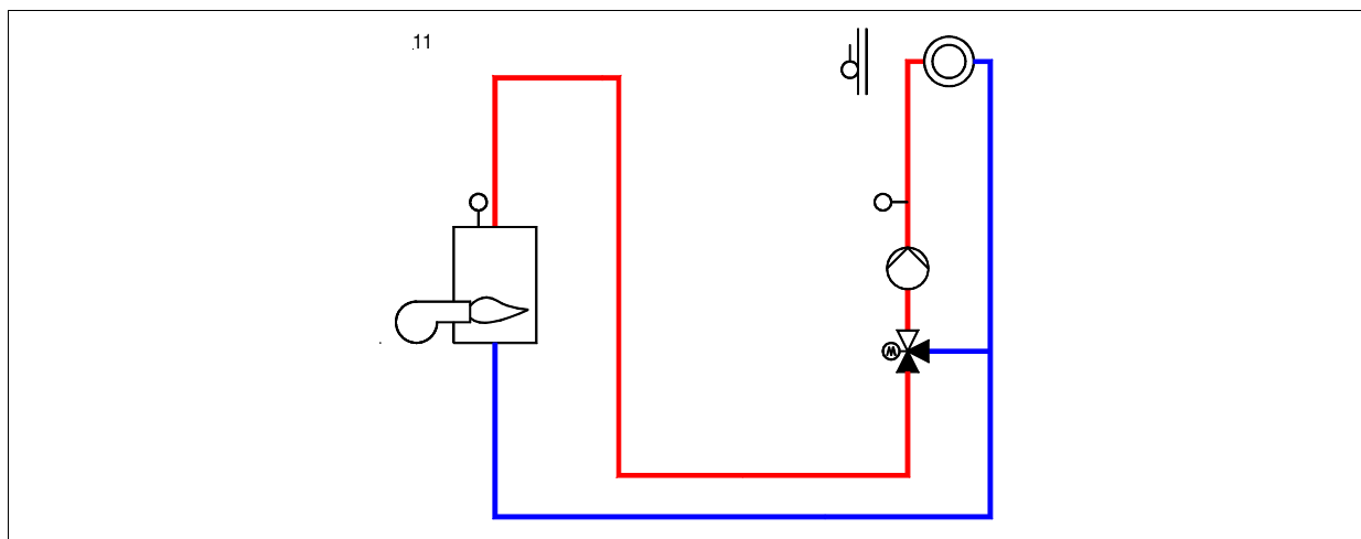
Schema 11: 1 Kessel (1-stufig), 1 gemischter Heizkreis
