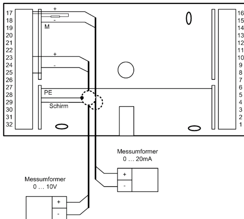
Abb. 10: Messumformer
