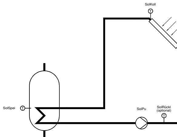
Abb. 43: Anlagentypen Brauchwasserkreis
