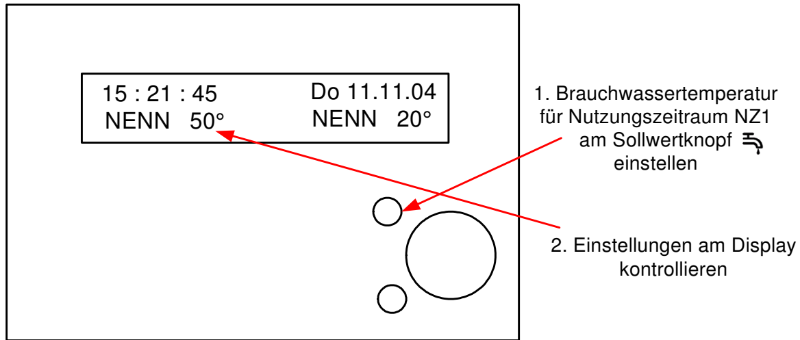
Abb. 30: Sollwertpoti Brauchwasserkreis
