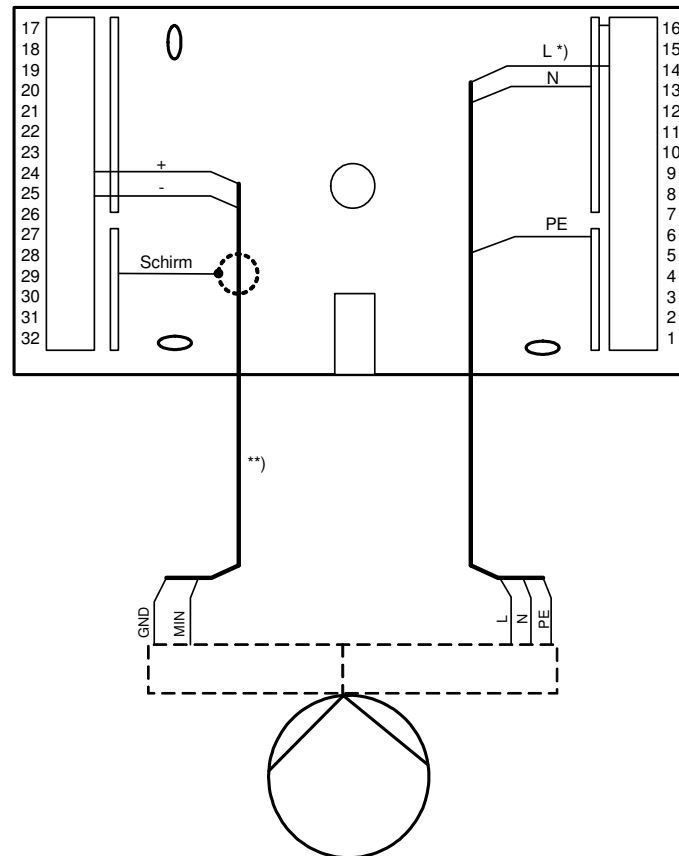
Abb. 14: Anschluss einer Pumpe (Beispiel)
