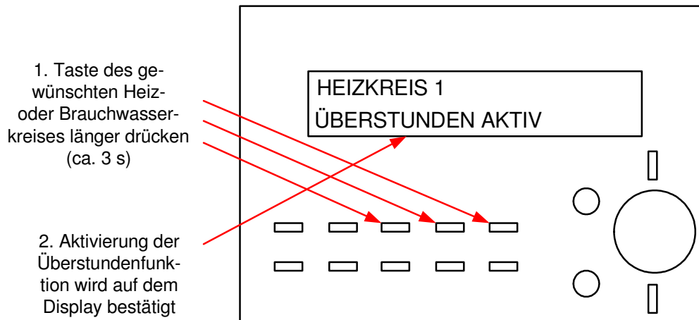
Abb. 33: Überstudentasten
