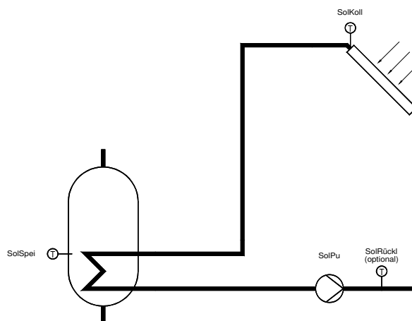
Abb. 43: Anlagentypen Brauchwasserkreis
