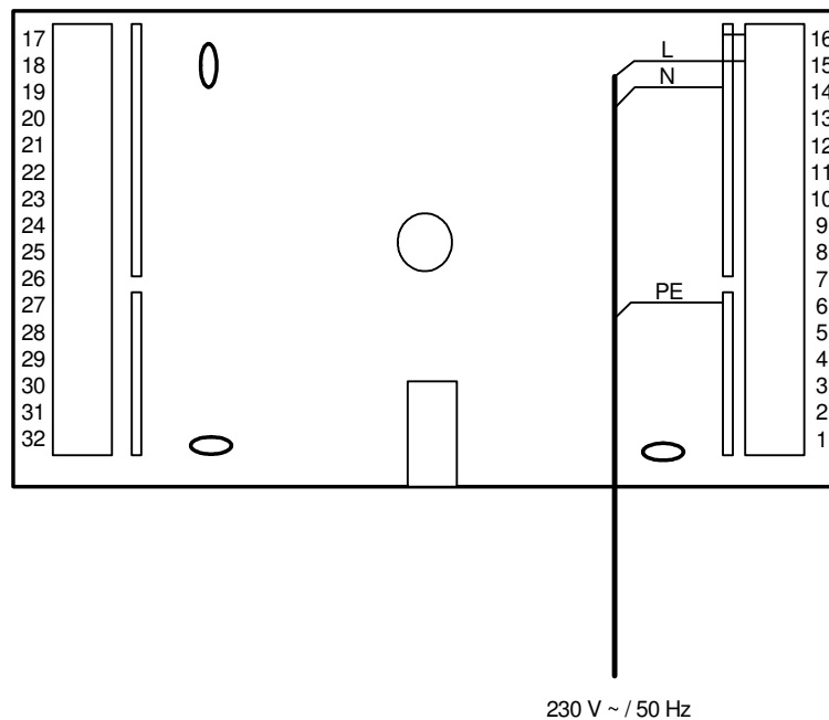
Abb. 8: Netzanschluss
