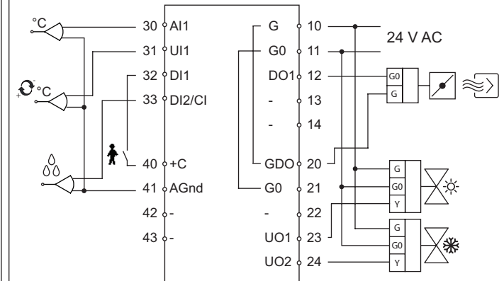
Abb. 4. Anschlussplan für RC
