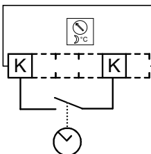
Abb. 7: Einschalten der Nachtabsenkungsfunktion.
