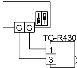
Figur 4: Omkopplare och anslutning vid rumsreglering med TG-R430 som extern givare och börvärde
