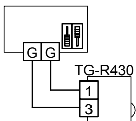
Abb. 4: Umschalter und Anschluß an Raumregelung mit TG-R430 als externen Fühler und Sollwert
