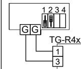
Figur 4 Omkopplarinställning och inkoppling vid rumsreglering med TG-R4xx som givare och börvärde.
