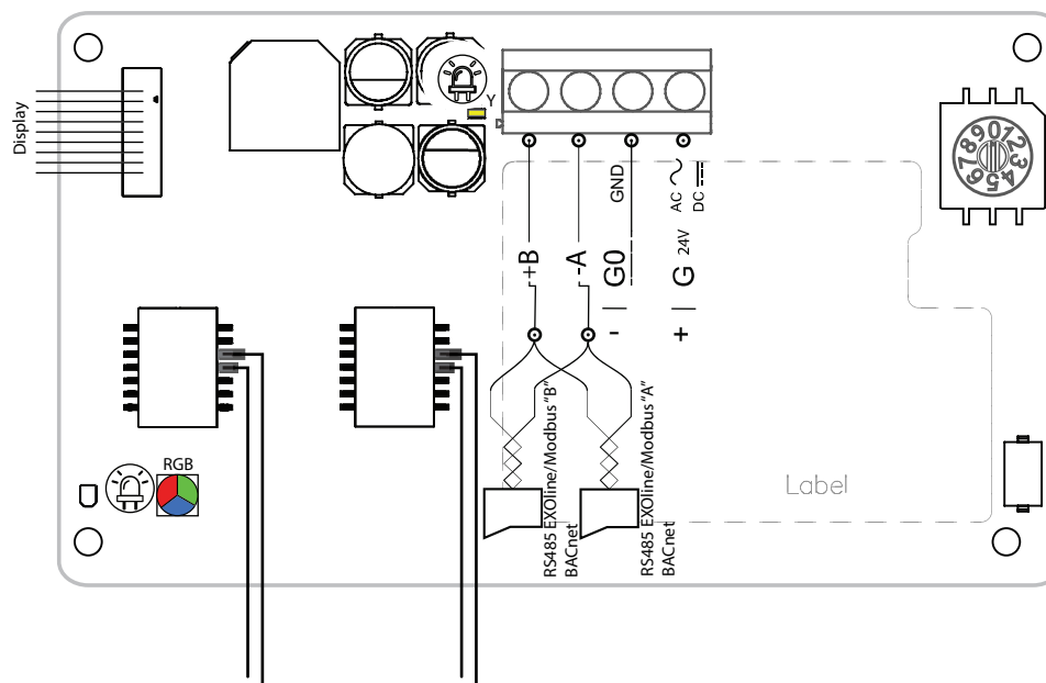
Bild C-3 Verdrahtungsbeispiel – PDTN-C
