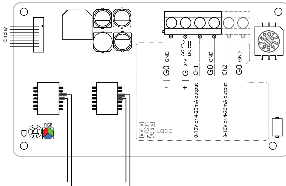
Bild C-2 Verdrahtungsbeispiel – PDTN
