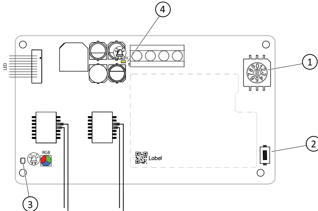
Bild 2-3 Leiterplatte (PCB)
