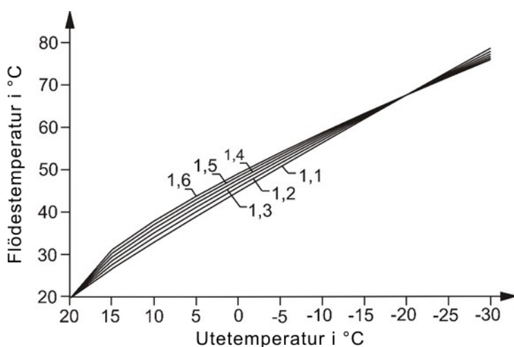
Figur 3-6 DIN-kurvans exponent
