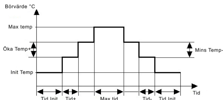
Figur 3-9 Betonghårdning
