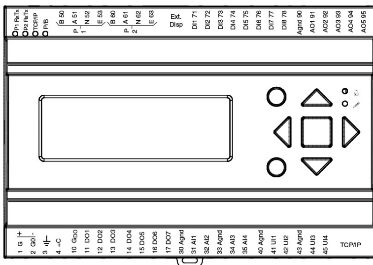
Figur 4-1 Plintpositioner 24 V modeller (Exigo Ardo)
