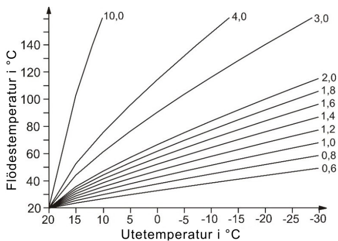
Figur 2-5 Lutning DIN-kurva
