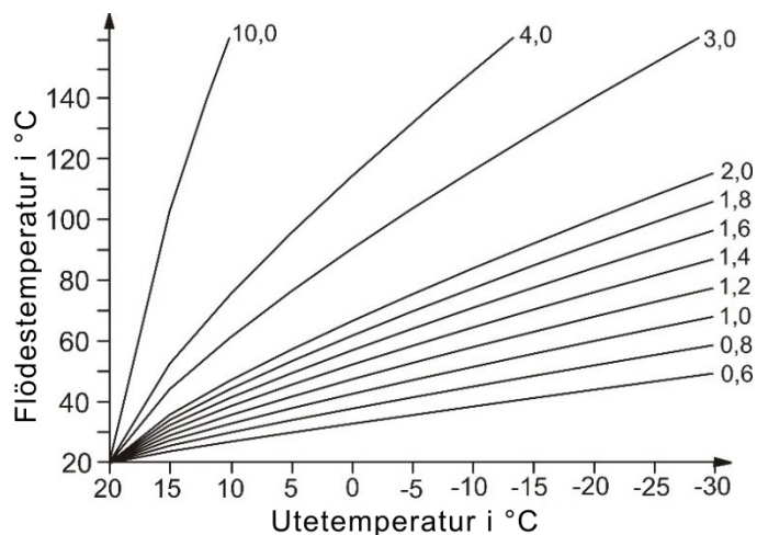
Figur 3-5 DIN-kurvans lutning
