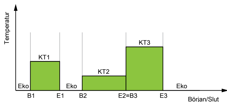
Figur 2-7 Tidsschema
