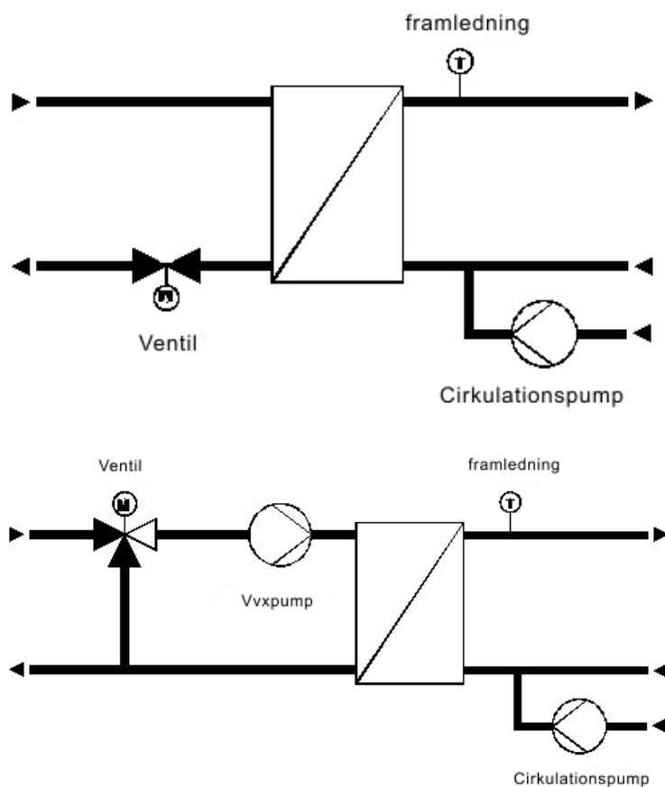
Figur 3-10 PI-styrd ventil för styrning av framledningstemperatur
