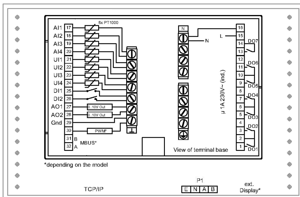
Figur 4-2 Plintpositioner 230 V modeller (Exigo Vido)
