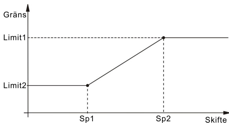
Figur 3-8 Variabel skiftningskurva
