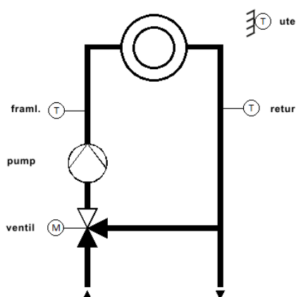
Figur 3-1 Blandad värmekrets
