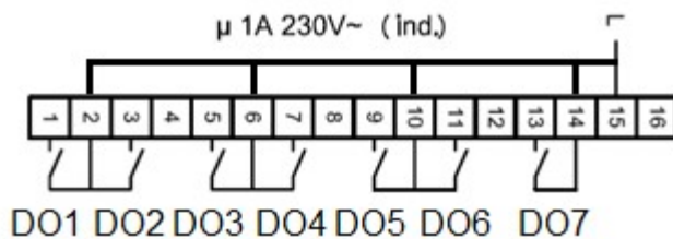
Figur 4-9 Digitala utgångar
