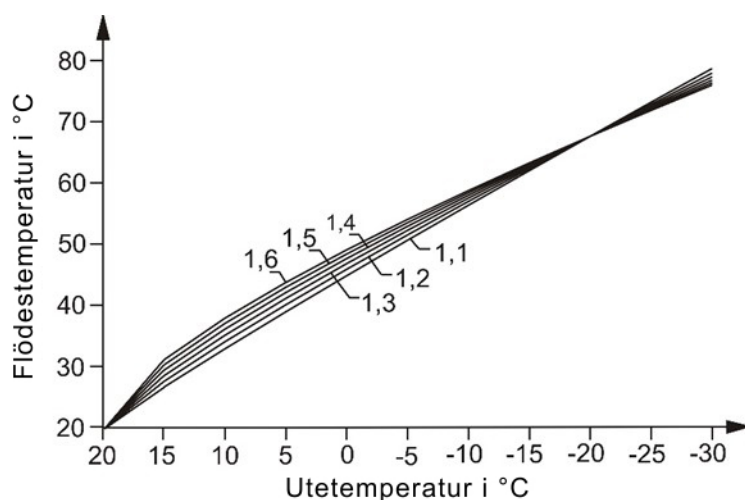
Figur 2-6 Exponent DIN-kurva
