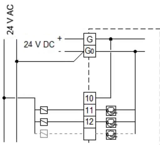
Figur 4-8 24 V DC-matning och 24 V AC-reläer
