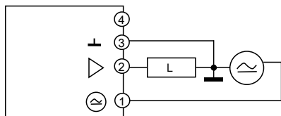
Kuva 1 Kytentäesimerkki (L= Vastus)
